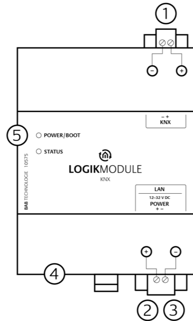
Abbildung 1: Anschlussbild
