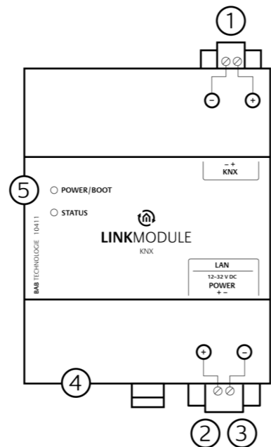
Abbildung 1: Anschlussbild
