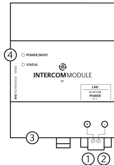
Abbildung 1: Anschlussbild
