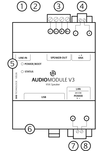
Abbildung 1: Anschlussbild
